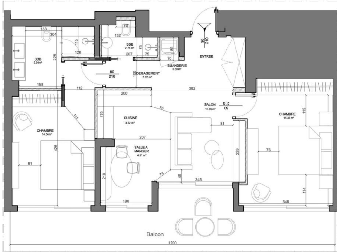
PLAN PROJET
